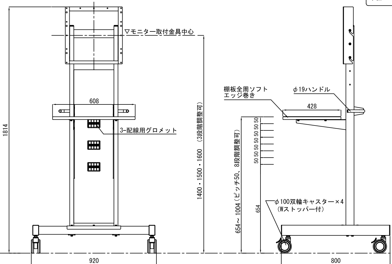
【正面図】
