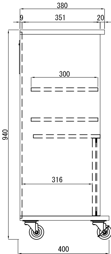
〔側面図（左側収納部）〕
