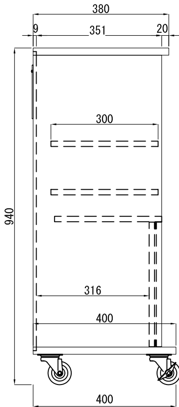
〔側面図（中央収納部）〕
